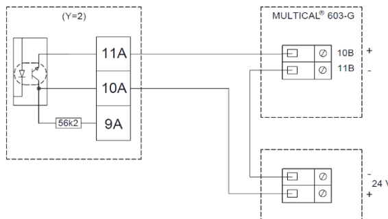
Рис. 36. Двухпроводное подключение передатчика импульсов с модулем выхода (Y=2) к MULTICAL® 603-G и внешним источником питания 24 В пост. тока 1) . Длина кабеля < 100 м.
