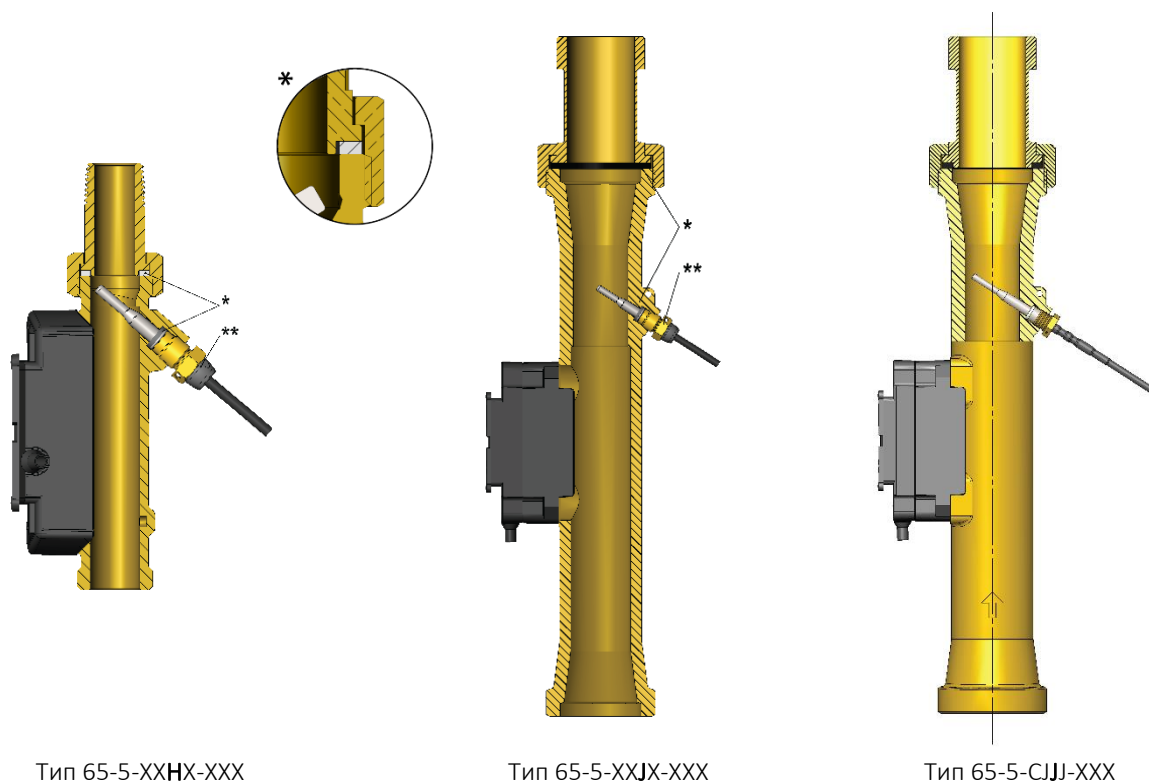
Рис. 14. Примеры датчиков расхода ULTRAFLOW® 54 (с резьбовым соединением) с датчиком TemperatureSensor 63 или коротким погружным датчиком DS38 мм (*Уплотнения; **Момент прибл. 4 Нм).
